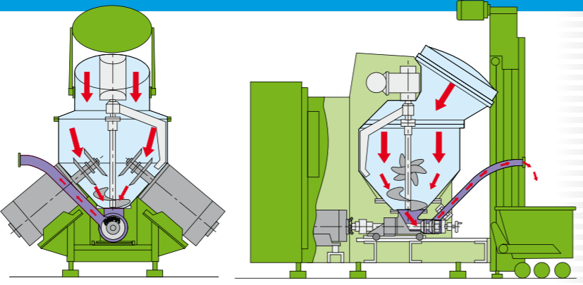
▼ Produktfließschema FD-Automaten Product flow system FD-Automats
